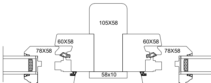
Assemblage sur chantier Renfort 105x58
