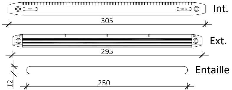
Grille d'entrée d'air 15/30m3/H Std
