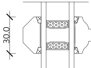
Petit bois collé intercalaire fictif
