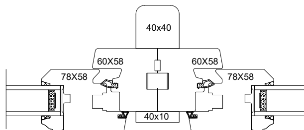
Assemblage sur chantier Renfort 40x40
