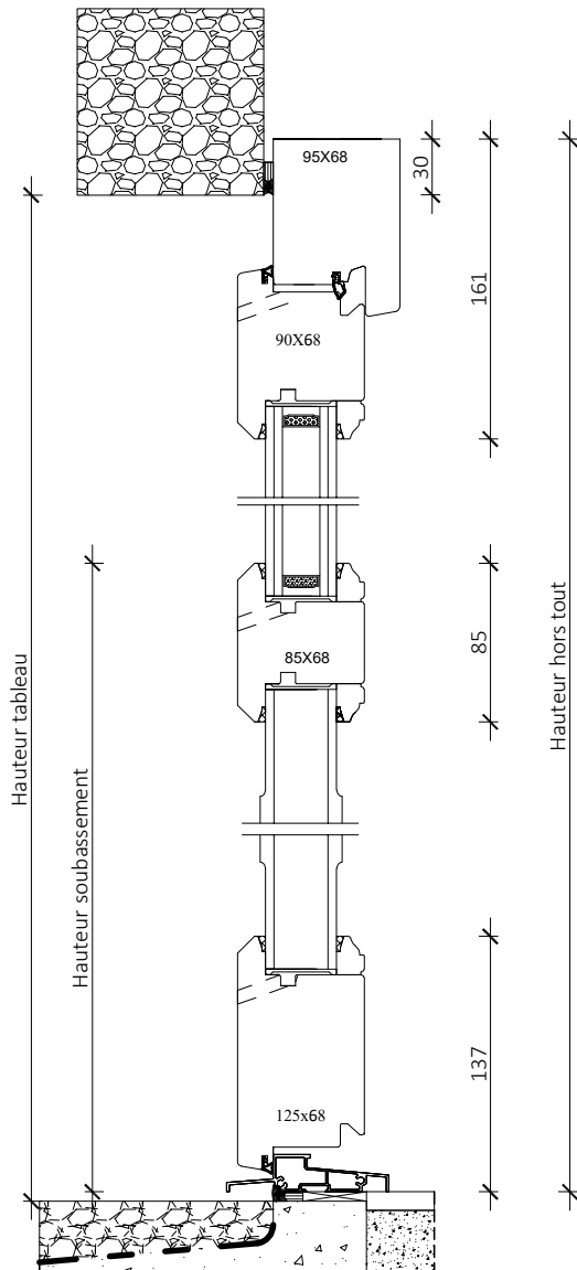
Coupe verticale
