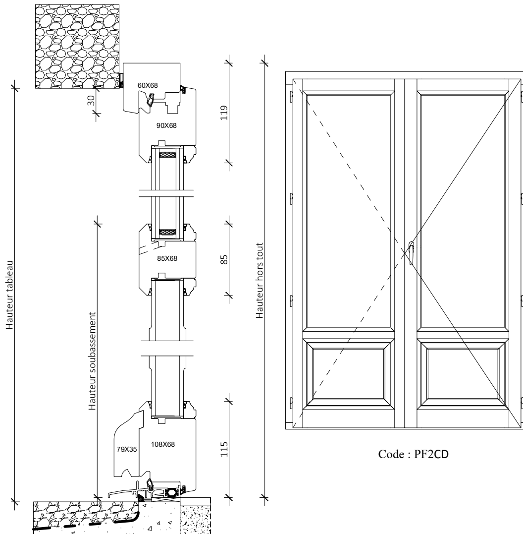
Coupe verticale
