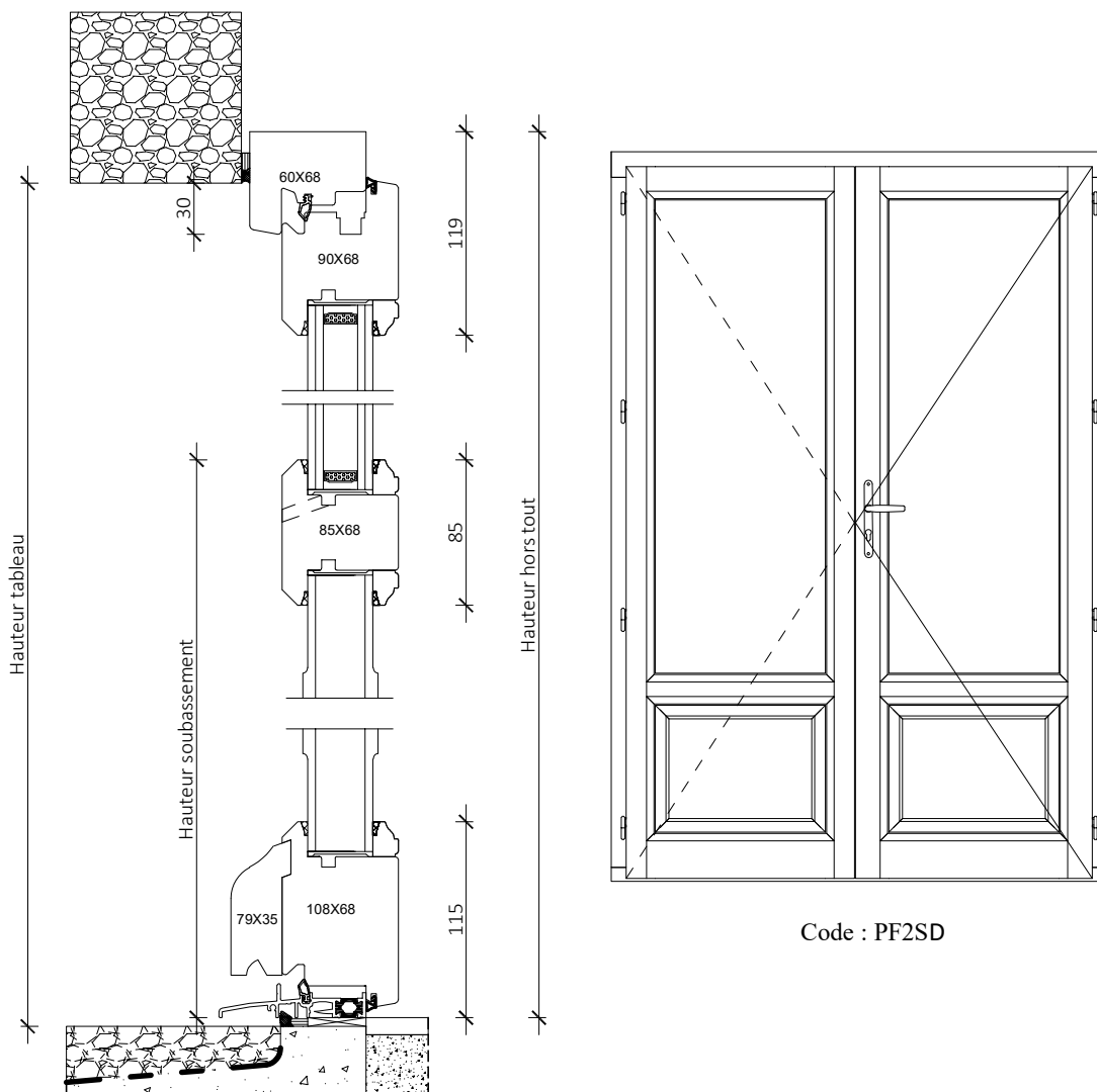
Coupe verticale
