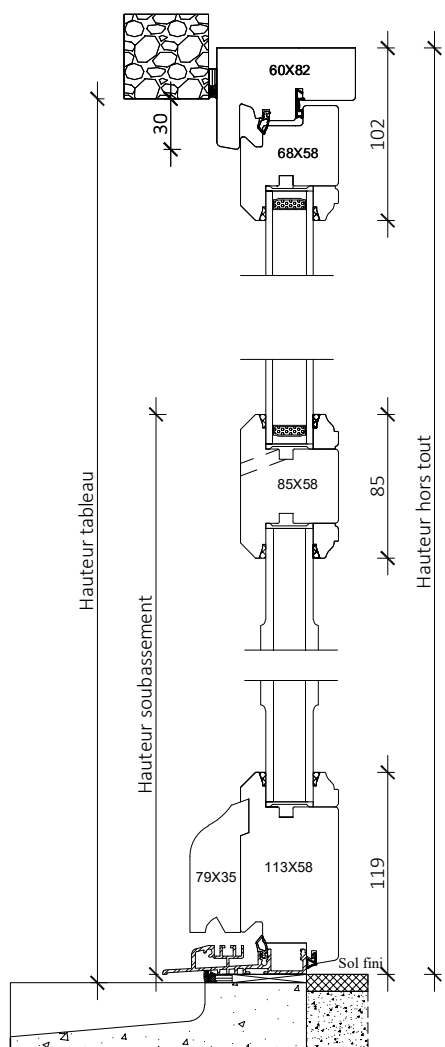
Coupe verticale
