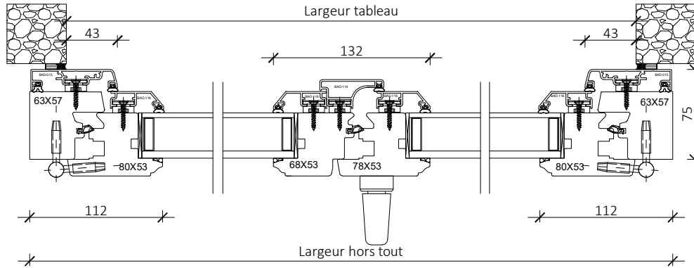
Coupe horizontale
