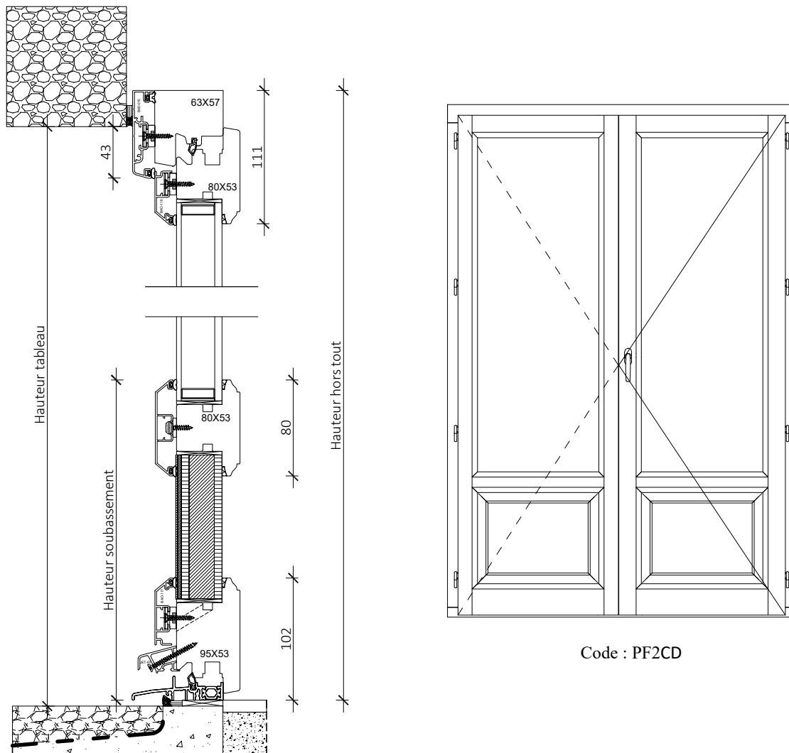
Coupe verticale
