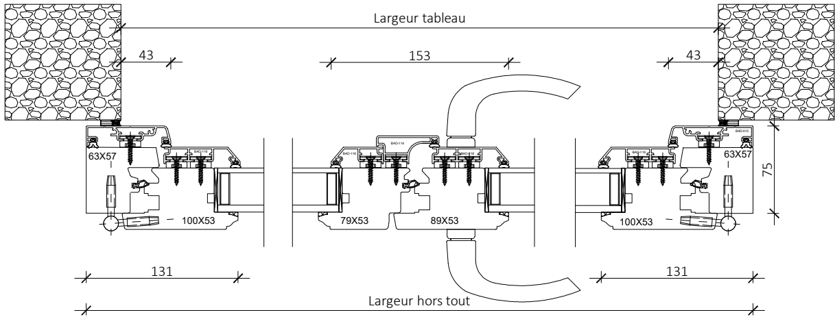
Coupe horizontale
