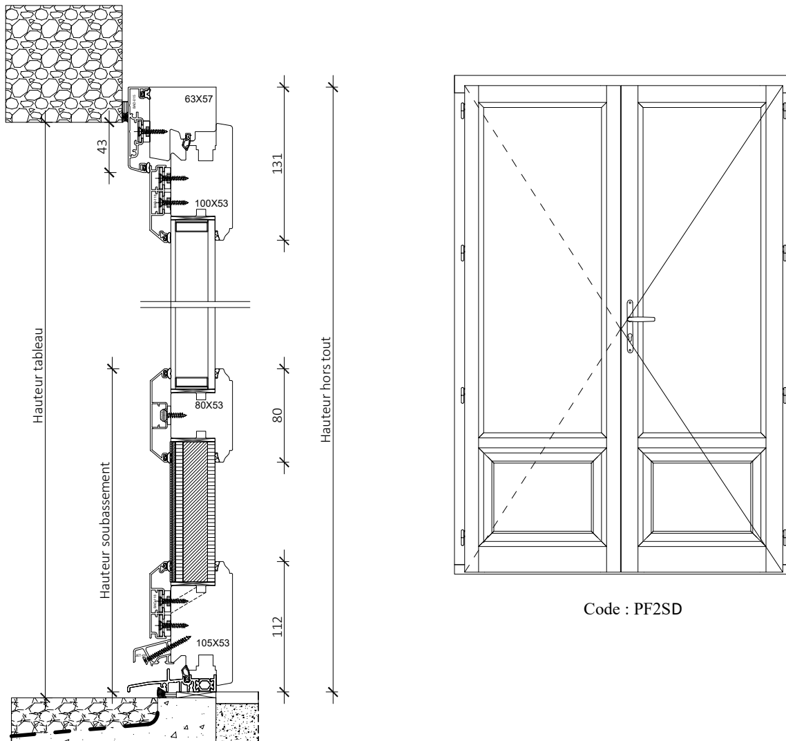
Coupe verticale
